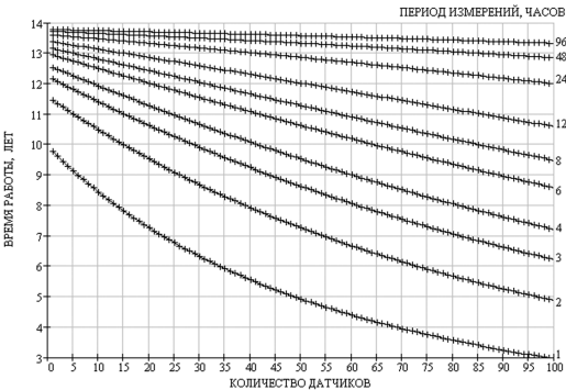
Рис.2. Расчетное время работы логгера ЛЦД-1/100-СД
