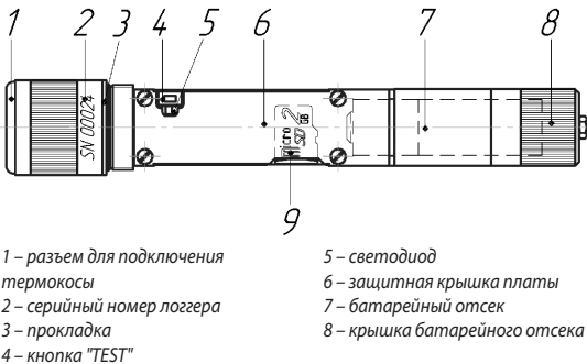
Рис.1. ЛЦД-1/100-СД без защитного кожуха
