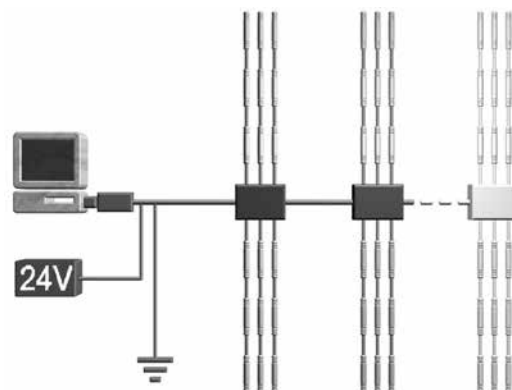
Конфигурация сети RS-485
